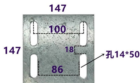
国标热镀锌 150*150*8
