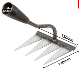
四齿耙
