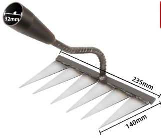
六齿耙
