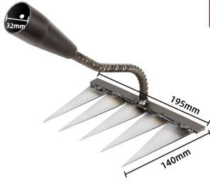
五齿耙
