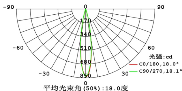
光曲线图 Light curve
